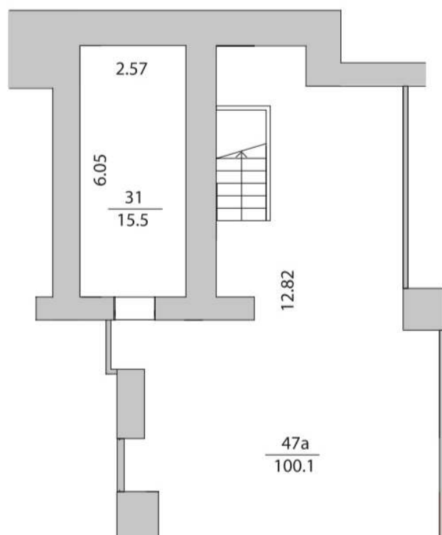
подвал
